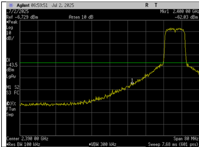
Low Ch_2419MHz_10MHz BW_-30dBc_Lower Band Edge Port 1
