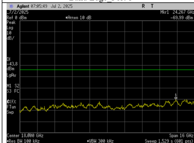
High Ch_2454MHz_10MHz BW_-30dBc_10- 26GHz_Port 1
