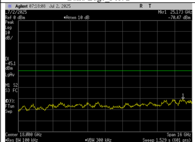
High Ch_2454MHz_10MHz BW_-30dBc_10- 26GHz_Port 2
