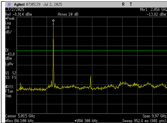
High Ch_2454MHz_10MHz BW_-30dBc_30MHz- 10GHz Port 1
