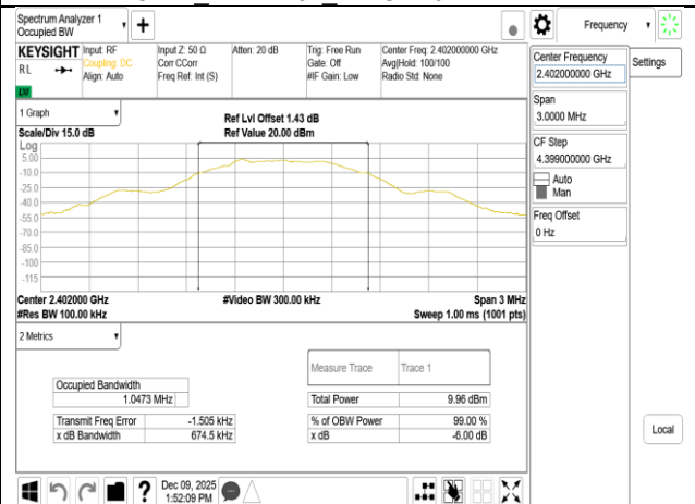
OBW_BLE 500k_LowCH00-2402MHz
