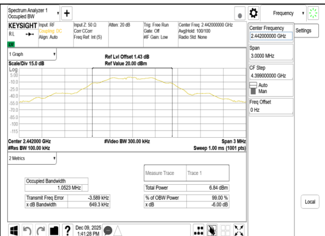
OBW_BLE 125k_MidCH20-2442MHz
