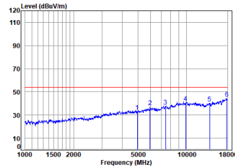
Dongle 2.4G SRD_2M_TX_CH_39_Horizontal-Avg
