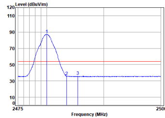
Dongle 2.4G SRD_2M_TX_CH_39_Vertical-Avg
