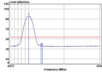
Dongle 2.4G SRD_1M_TX_CH_39_Horizontal-Avg
