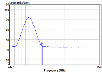
Dongle 2.4G SRD_2M_TX_CH_39_Horizontal-Avg
