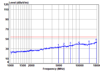
Dongle 2.4G SRD_1M_TX_CH_39_Vertical-Avg
