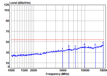
Dongle 2.4G SRD_1M_TX_CH_39_Horizontal-Avg
