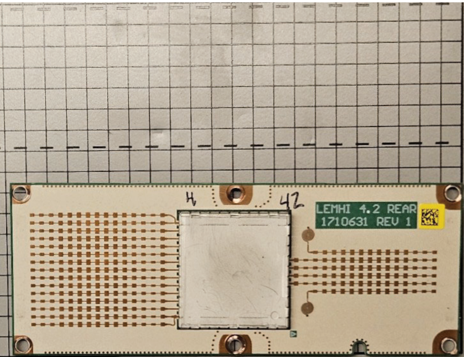
TX Antenna Array
