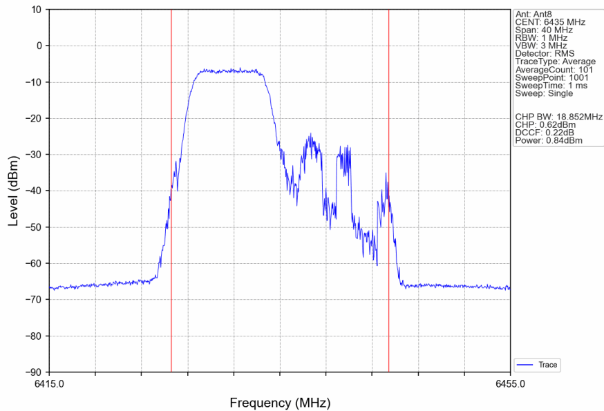
802.11be(EHT20)_LCH_6435MHz_26+52_ / Ant8_NTNV
