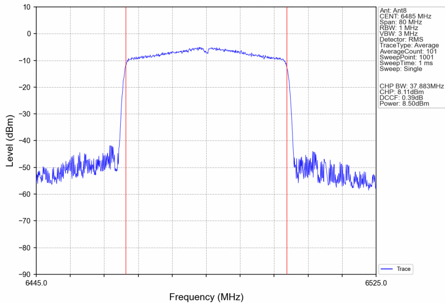
802.11be(EHT40)_MCH_6485MHz_RU484_Left_Ant8_NTNV
