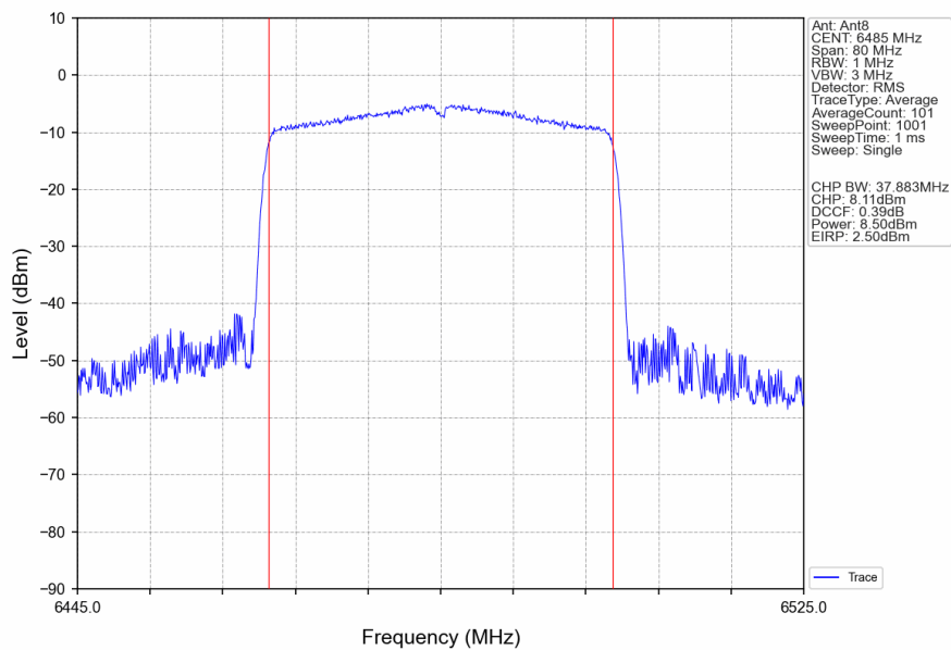
802.11be(EHT40)_MCH_6485MHz_RU484_Left_Ant8_NTNV
