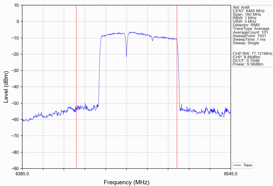
802.11be(EHT80)_LCH_6465MHz_242+484 / Ant8_NTNV
