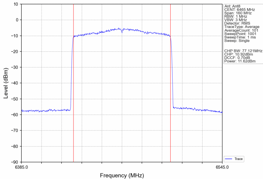
802.11be(EHT80)_LCH_6465MHz_RU996_Left_Ant8_NTNV
