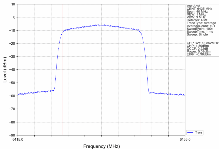
802.11be(EHT20)_LCH_6435MHz_RU242_Left_Ant8_NTNV
