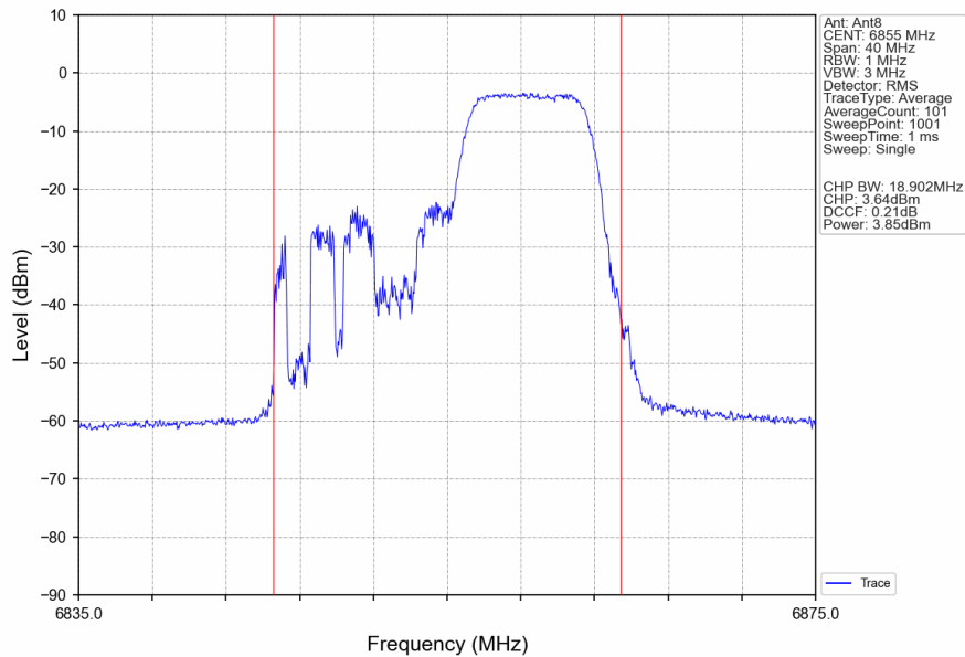
802.11be(EHT20)_HCH_6855MHz_26+52_ / Ant8_NTNV
