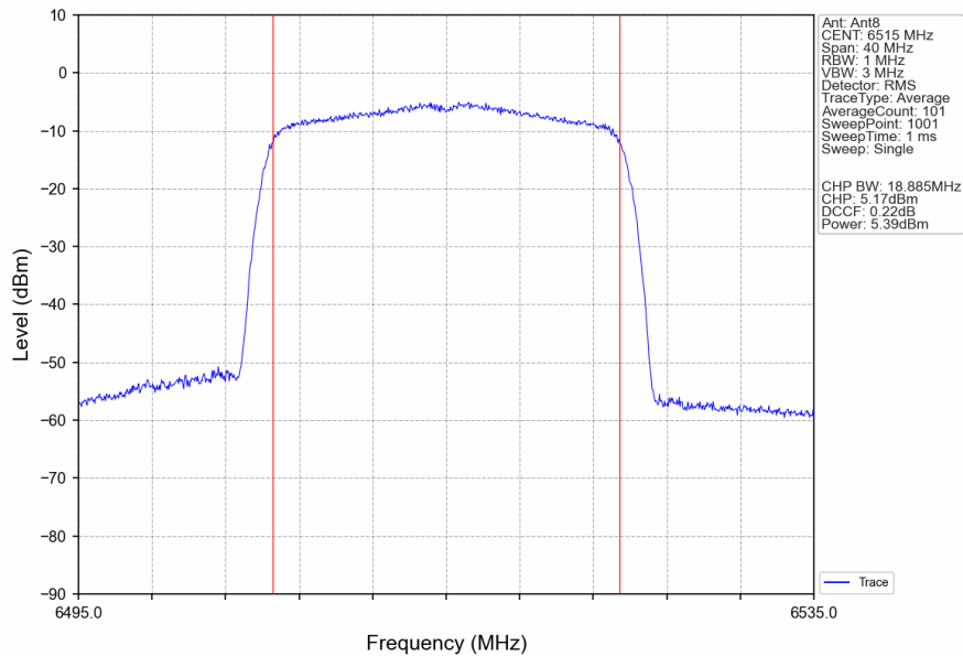
802.11be(EHT20)_HCH_6515MHz_RU242_Left_Ant8_NTNV
