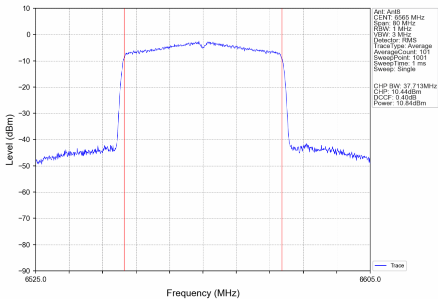
802.11be(EHT40)_LCH_6565MHz_RU484_Left_Ant8_NTNV
