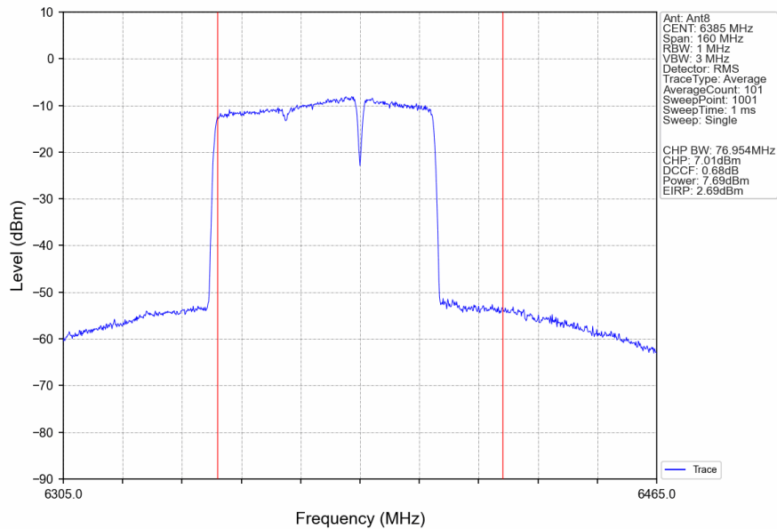
802.11be(EHT80)_HCH_6385MHz_242+484 / Ant8_NTNV
