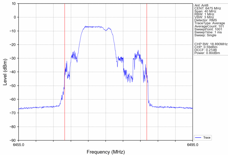
802.11be(EHT20)_MCH_6475MHz_26+52_ / Ant8_NTNV
