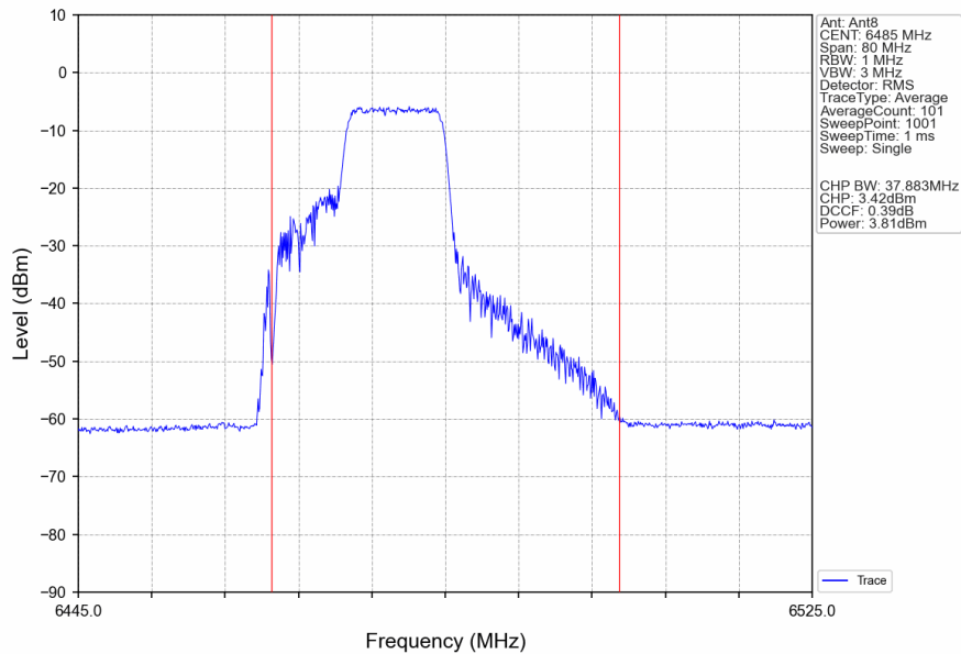
802.11be(EHT40)_MCH_6485MHz_26+106_/_Ant8_NTNV
