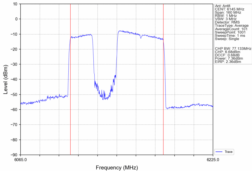
802.11be(EHT80)_MCH_6145MHz_242+484 / Ant8_NTNV
