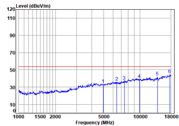
2.4G SRD_1M_TX_CH_39_Vertical-Avg
