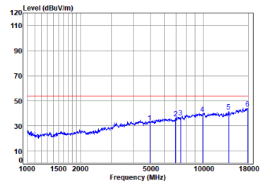
2.4G SRD_2M_TX_CH_39_Horizontal-Avg
