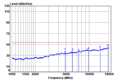
2.4G SRD_2M_TX_CH_19_Vertical-Avg
