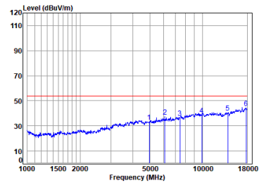
2.4G SRD_1M_TX_CH_39_Horizontal-Avg
