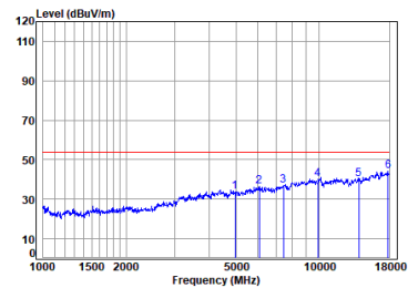
2.4G SRD_2M_TX_CH_39_Vertical-Avg
