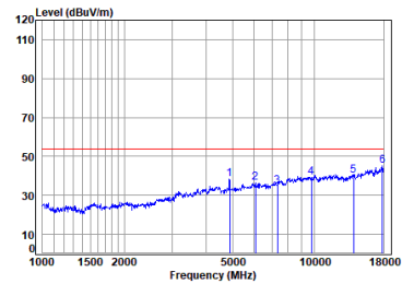
2.4G SRD_1M_TX_CH_19_Horizontal-Avg
