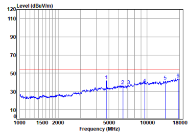
2.4G SRD_2M_TX_CH_00_Horizontal-Avg
