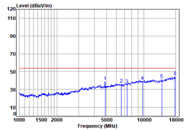
2.4G SRD_2M_TX_CH_19_Horizontal-Avg
