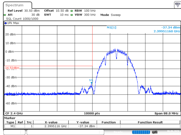
802.11b_2412MHz
