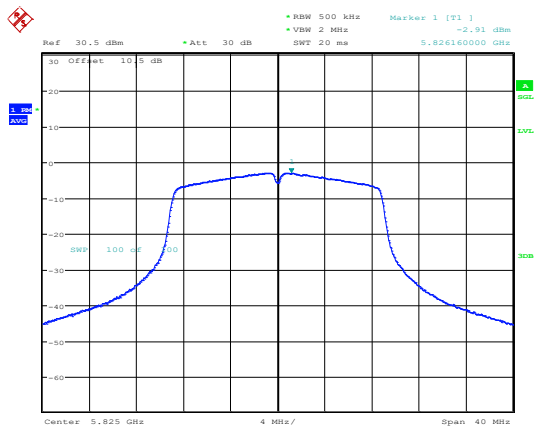
802.11ac20_5825MHz_Chain 1
