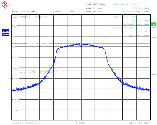
802.11ac20_5580MHz_Chain 0
