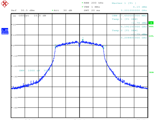
802.11ac20_5200MHz_Chain 0
