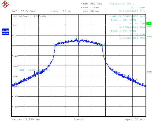
802.11ac20_5785MHz_Chain 0
