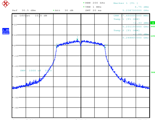
802.11ac20_5240MHz_Chain 0
