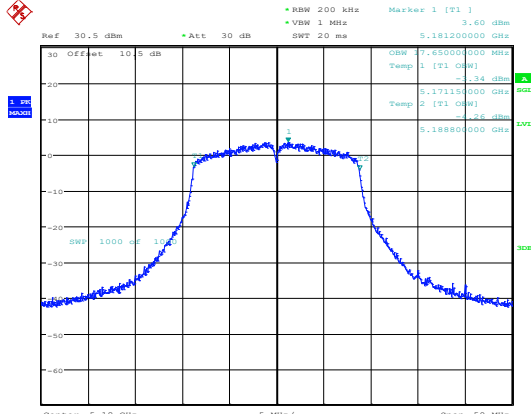
802.11ac20_5180MHz_Chain 0
