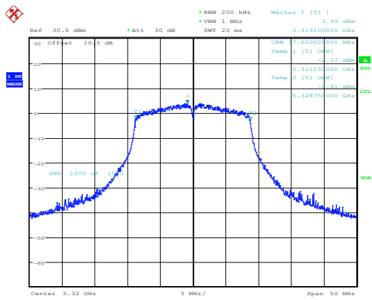
802.11ac20_5320MHz_Chain 0
