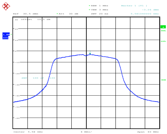
802.11ac20_5580MHz_Chain 1
