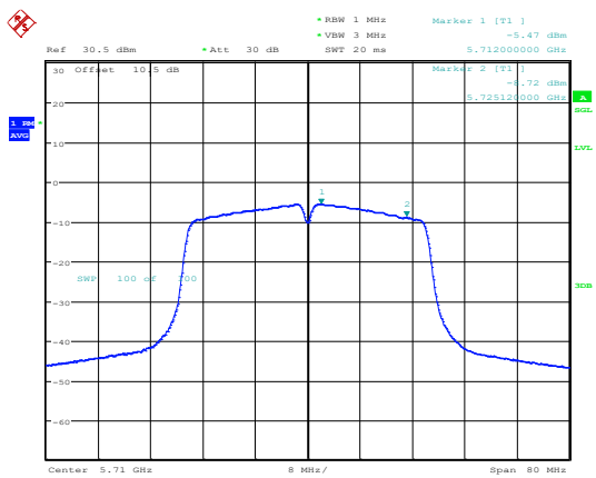
802.11ac40_5710MHz_Chain 1
