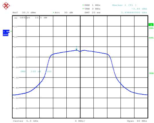
802.11ac20_5500MHz_Chain 1
