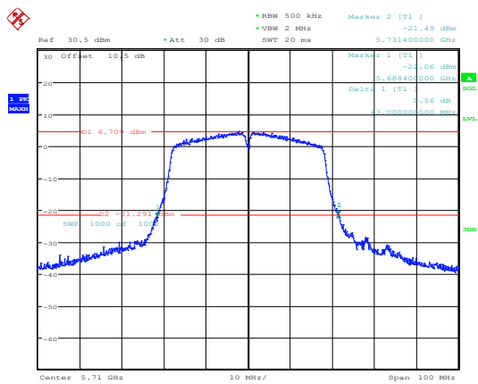
802.11ac40_5710MHz_Chain 0
