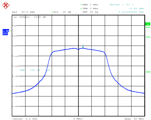
802.11a_5500MHz_Chain 1
