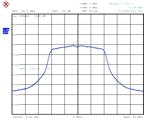
802.11a_5320MHz_Chain 1
