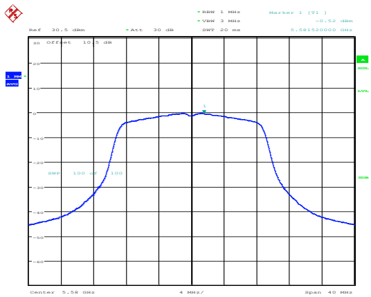
802.11ac20_5580MHz_Chain 0
