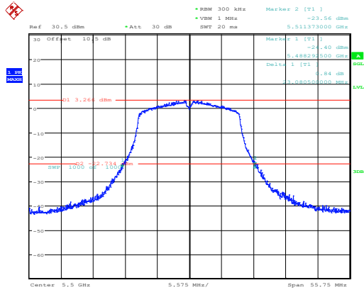
802.11ac20_5500MHz_Chain 0
