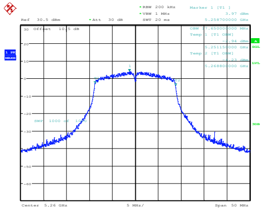
802.11ac20_5260MHz_Chain 0
