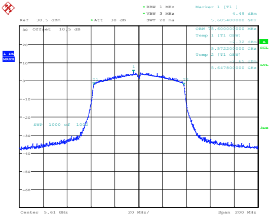
802.11ac80_5610MHz_Chain 0
