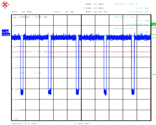
802.11ac20_5200MHz_Chain 0
