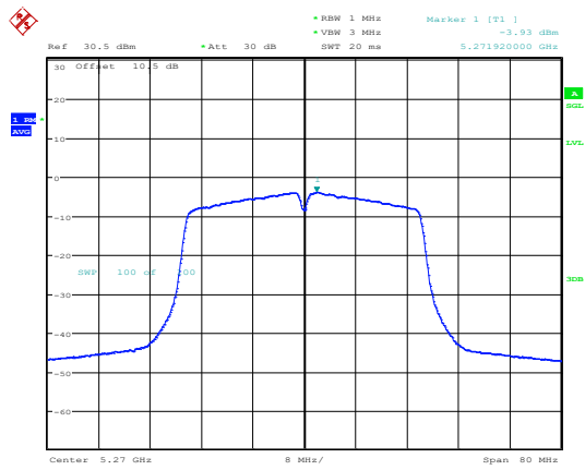
802.11ac40_5270MHz_Chain 1
