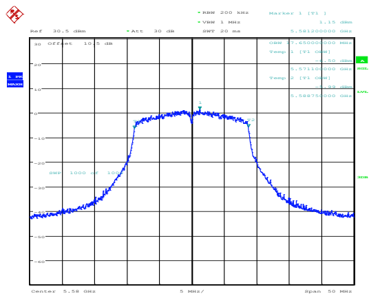
802.11ac20_5580MHz_Chain 0
