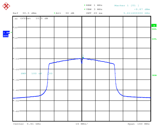
802.11ac80_5610MHz_Chain 1
