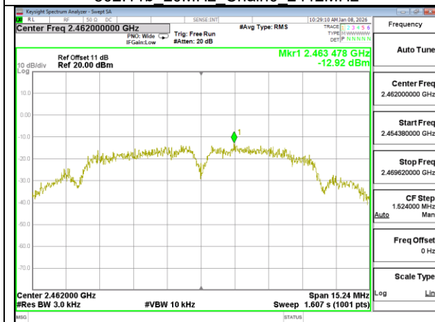
802.11b 20MHz Chain0 2462MHz
