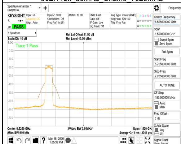
802.11ax 80MHz Chain1 6145MHz
