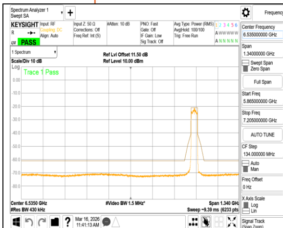
802.11ax 40MHz Chain0 6925MHz
