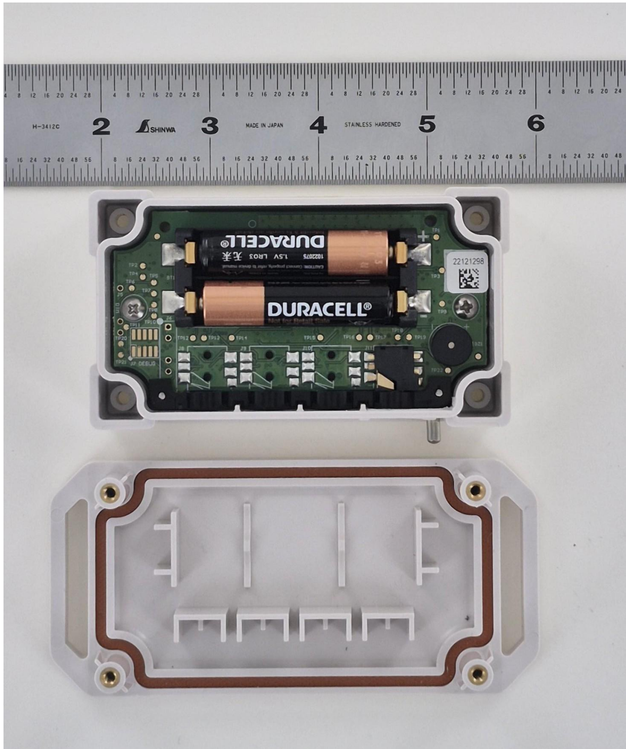
MX1104 Battery Door & PCB Back
