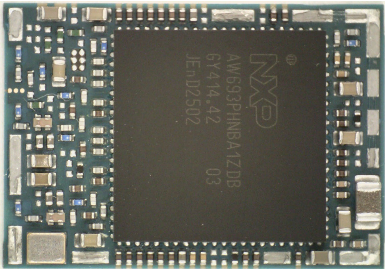
JODY-W683-01A_internal photo.jpg
