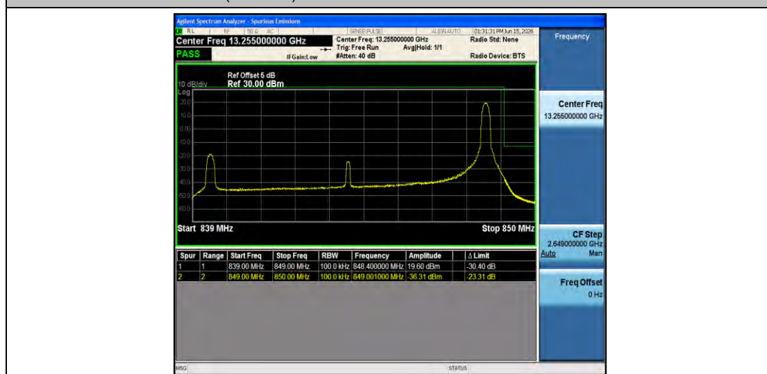
26(824-849)-10MHz-QPSK-26990-1RB#49-PASS
