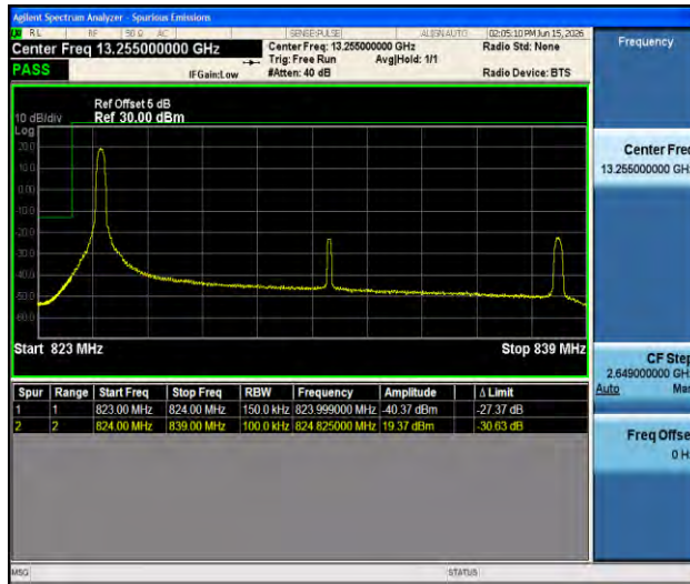
26(824-849)-15MHz-QPSK-26865-1RB#0-PASS
