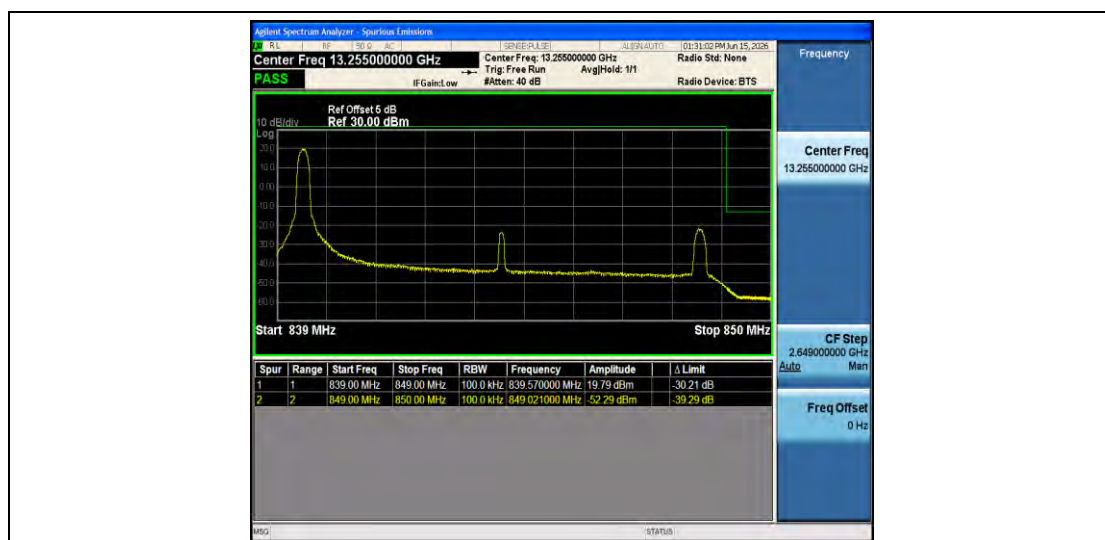
26(824-849)-10MHz-QPSK-26990-1RB#0-PASS
