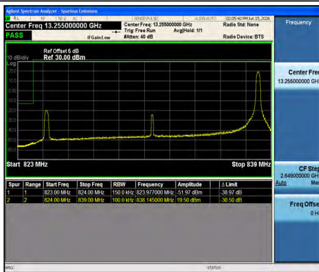
26(824-849)-15MHz-QPSK-26865-1RB#74-PASS
