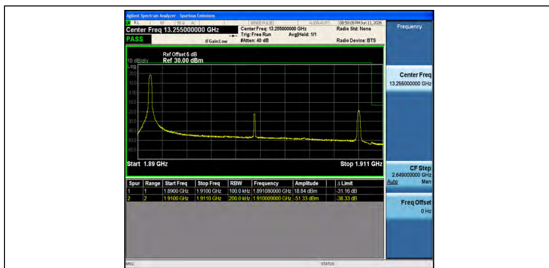
Band2-20MHz-QPSK-19100-1RB#0-PASS
