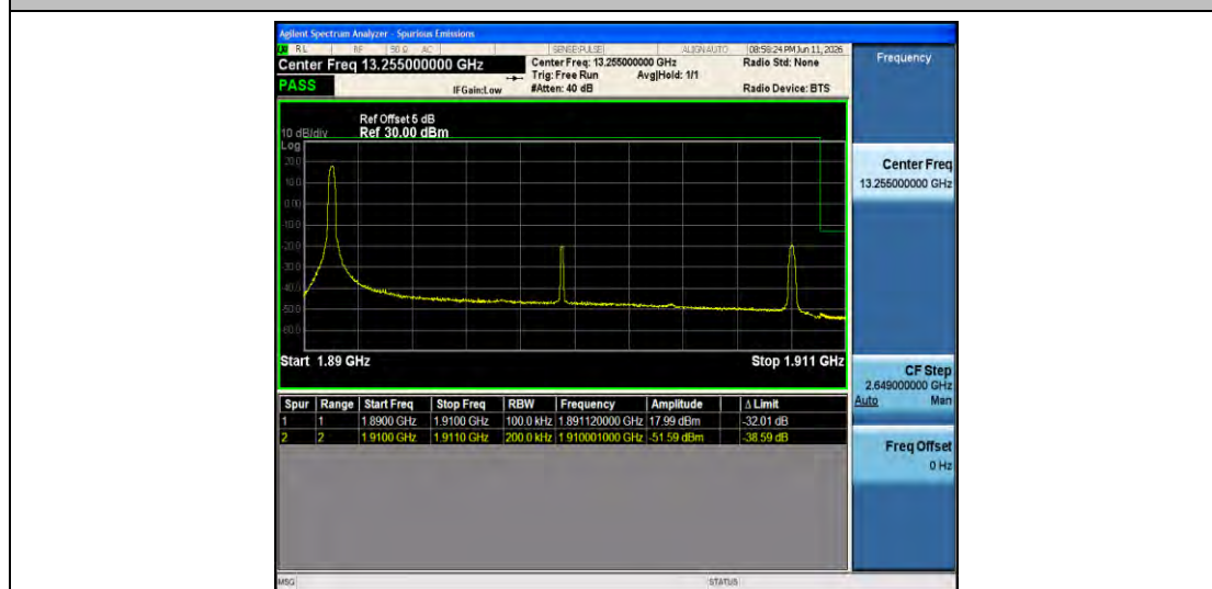
Band2-20MHz-16QAM-19100-1RB#0-PASS
