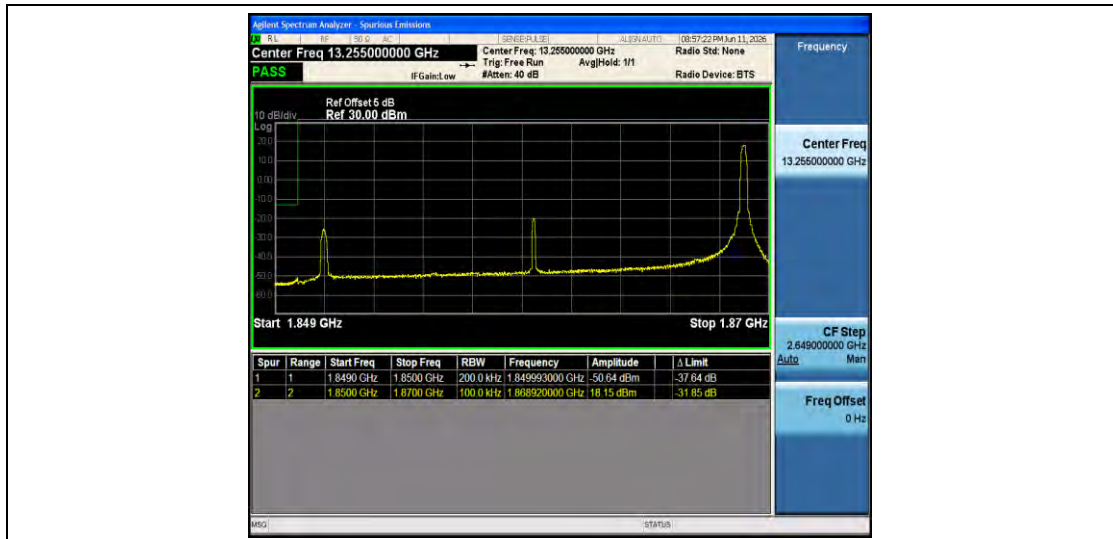
Band2-20MHz-16QAM-18700-1RB#99-PASS
