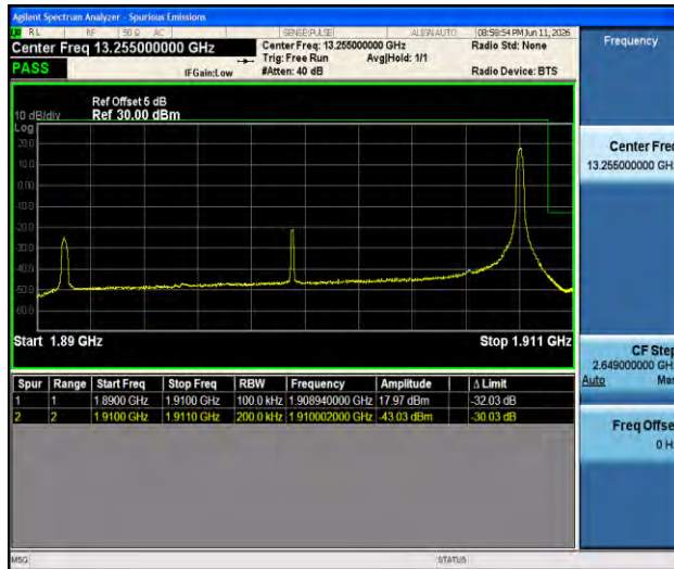
Band2-20MHz-16QAM-19100-1RB#99-PASS
