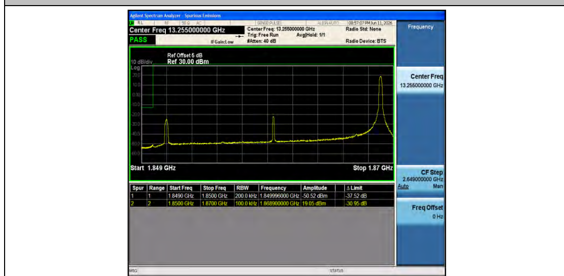
Band2-20MHz-QPSK-18700-1RB#99-PASS
