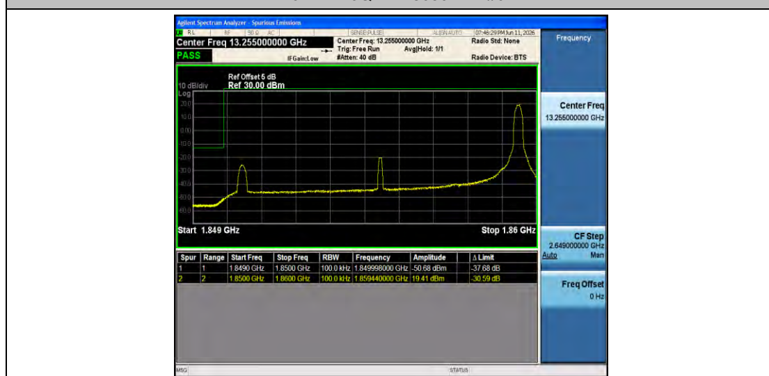
Band2-10MHz-QPSK-18650-1RB#49-PASS
