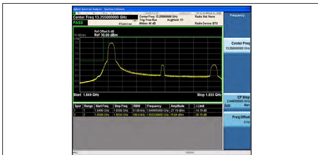
Band2-5MHz-QPSK-18625-1RB#0-PASS
