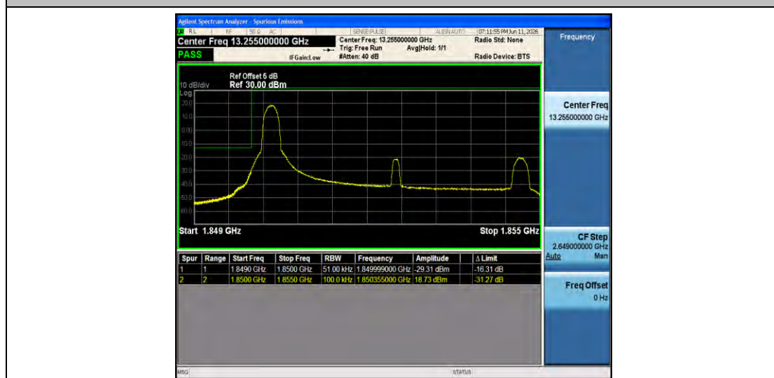
Band2-5MHz-16QAM-18625-1RB#0-PASS
