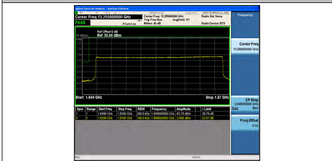
Band2-20MHz-16QAM-18700-100RB#0-PASS
