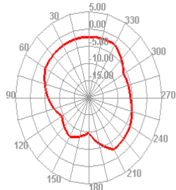
2500.000MHz H
