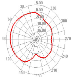
2500.000MHz
