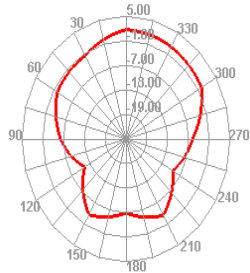
2450.000MHz H
