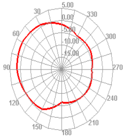
2400.000MHz E1
