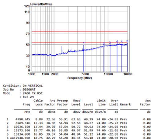
BLE_2M_TX_CH_39_Vertical
