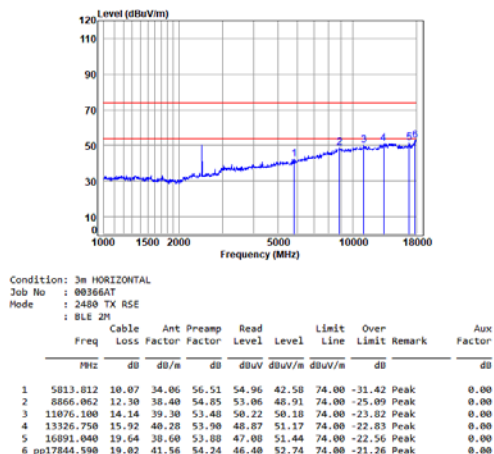
BLE_2M_TX_CH_39_Horizontal
