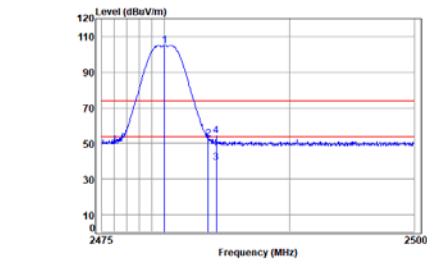
BLE_2M_TX_CH_39_Horizontal
