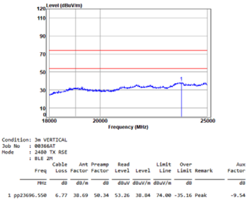
BLE_2M_TX_CH_39_Vertical
