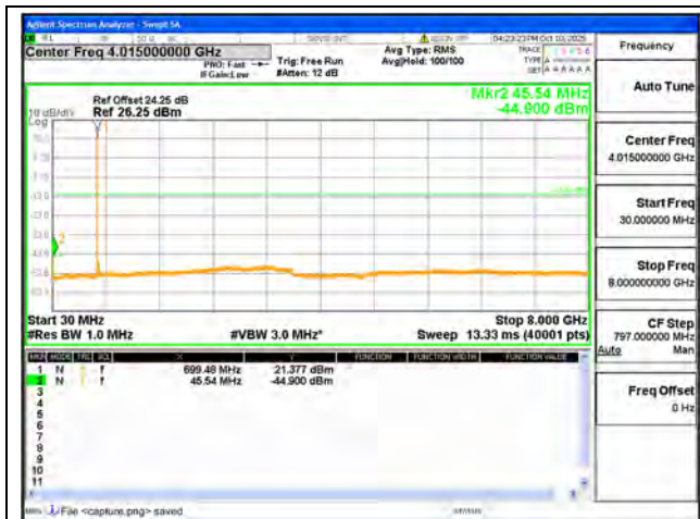
B12 / 1.4MHz / Low CH / QPSK
