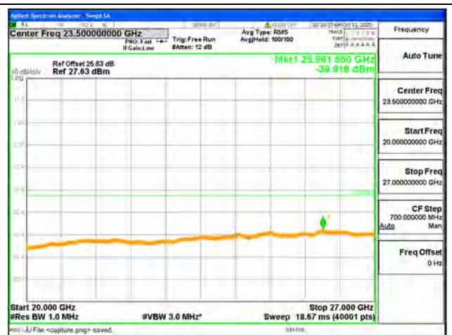
B41-20G-27G / 10MHz / Low CH / QPSK
