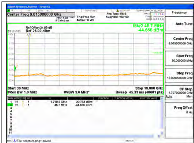
B66 / 1.4MHz / Low CH / QPSK
